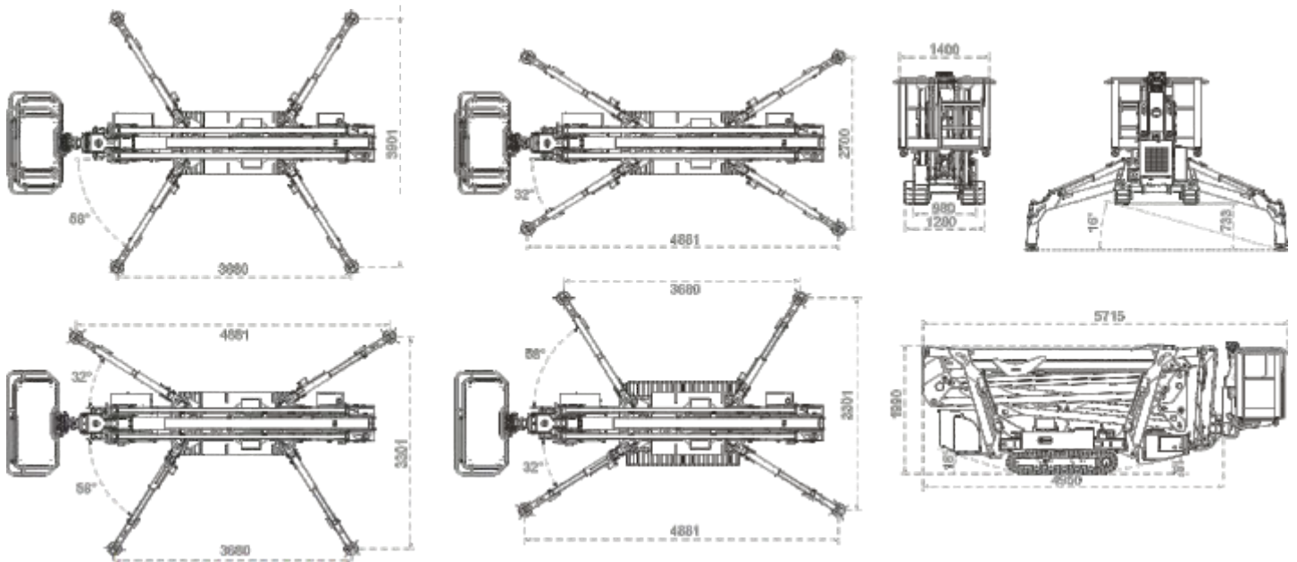
Lungime brat 12 m cu greutate laterala de 140 kg cu inaltimea articulatiei de 9 m.
